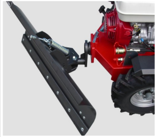
Lame de déneigement
