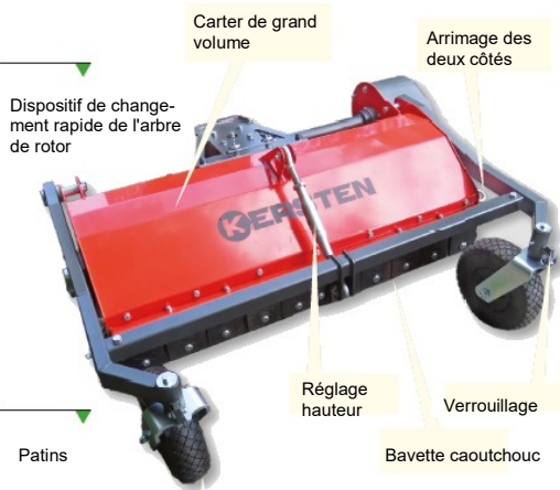
Verrouillage des roues (pour travail sur des pentes)
