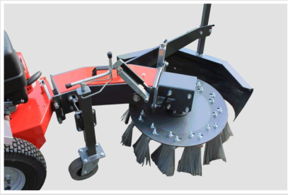
Brosse de désherbage
